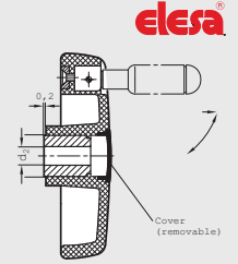
Elesa Model ESW + IR
