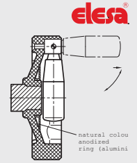
Elesa Model VDO.FP + IR
