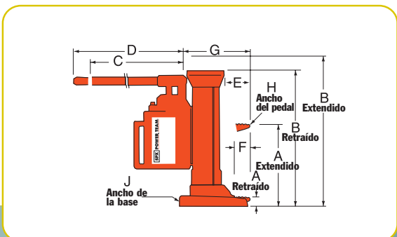
El gato de uña de la serie J es un gato extremadamente robusto utilizado para reparar carretillas elevadoras.
