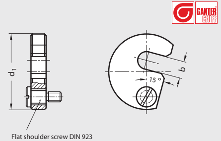
Flat shoulder screw DIN 923
