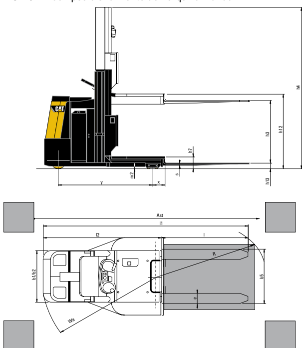
NOL10NV: con posicionamiento de horquilla manual
